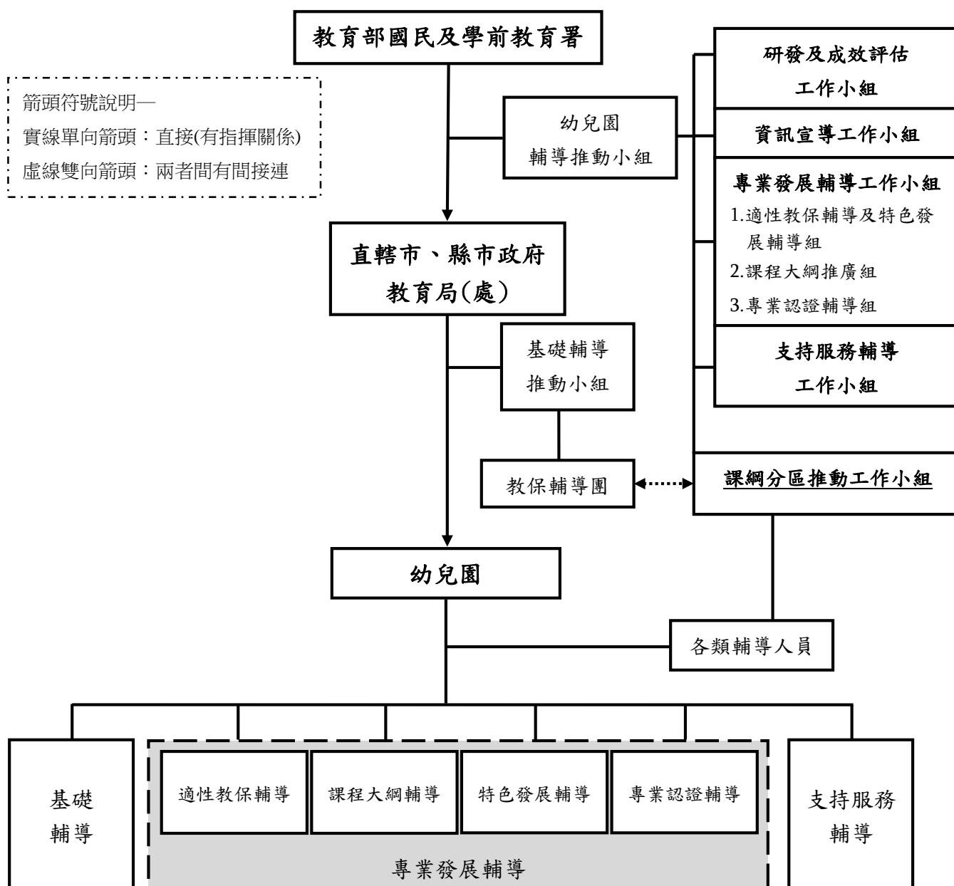
圖 1 輔導網路圖
