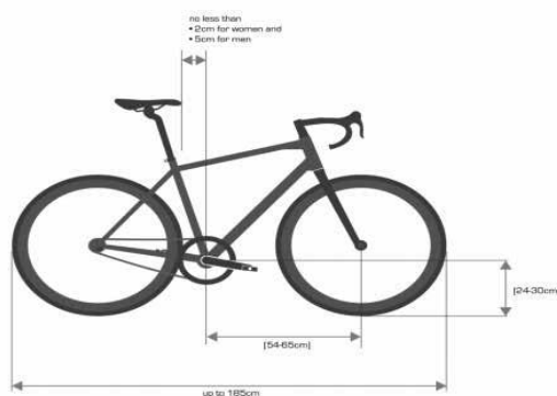
圖二、車架設定規定圖
